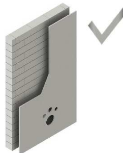
Duvarönü alçıpan kaplama uygulaması
