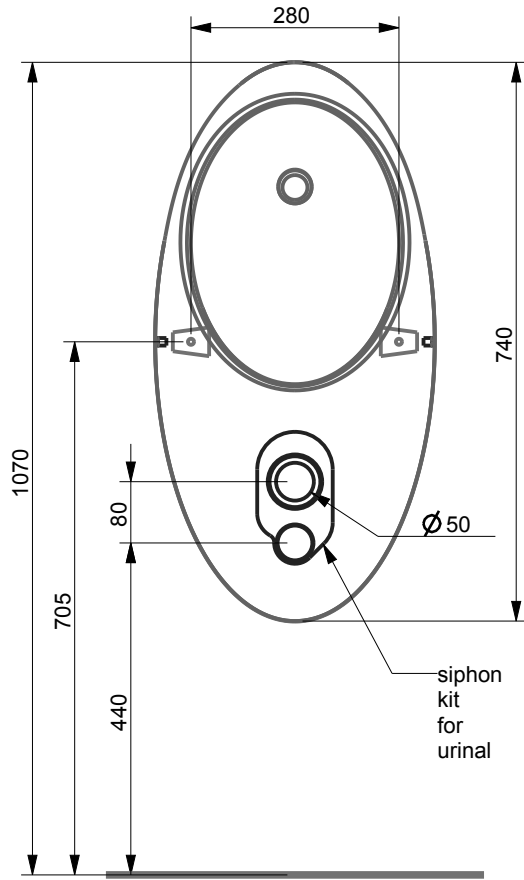
ÖN / FRONT
