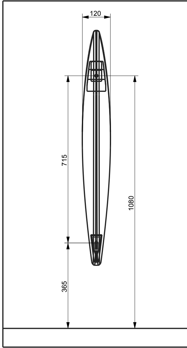
ÖN / FRONT
