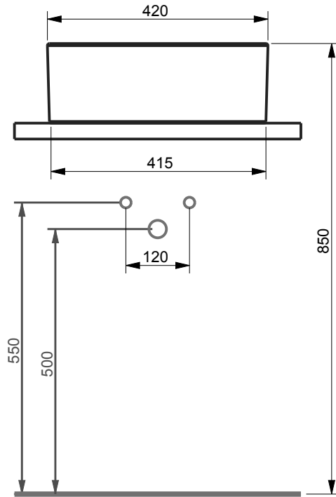
ÖN / FRONT
