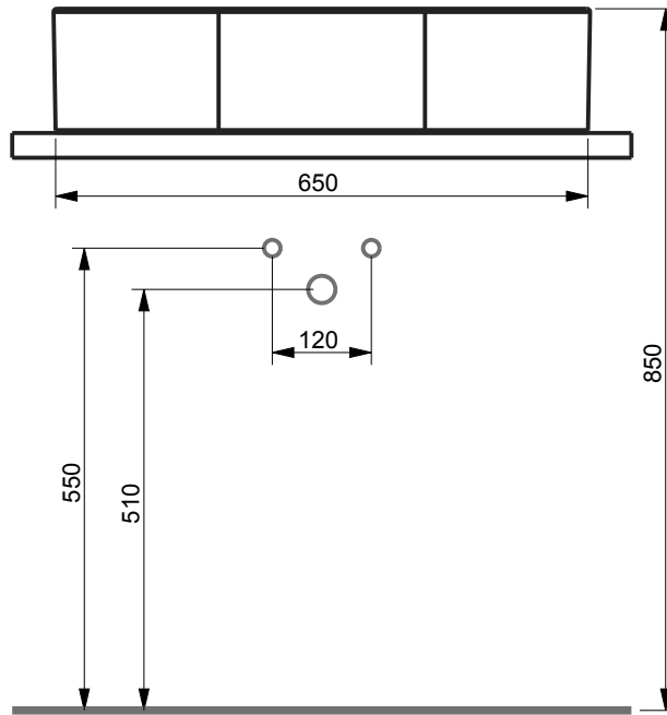
ÖN / FRONT
