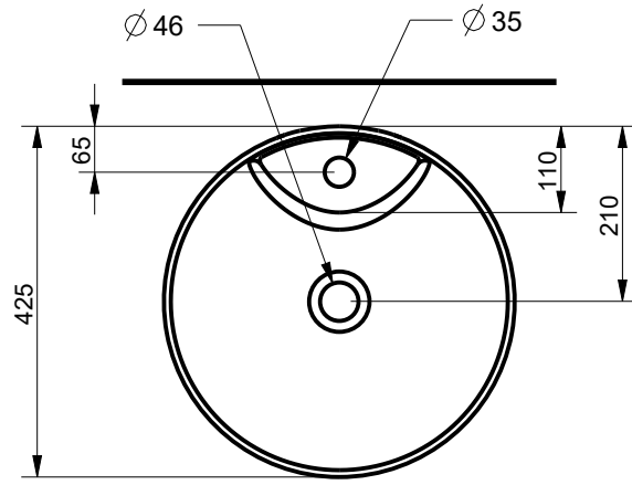
ÜST / TOP
