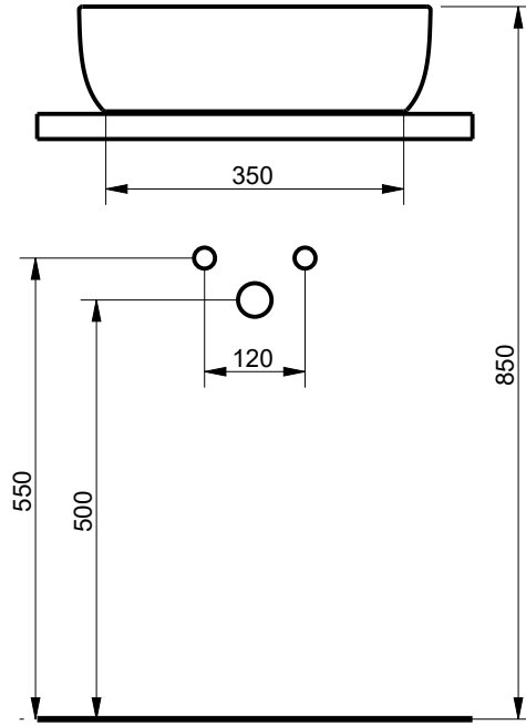
ÖN / FRONT
