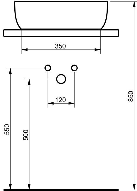
ÖN / FRONT
