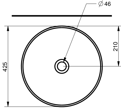
ÜST / TOP
